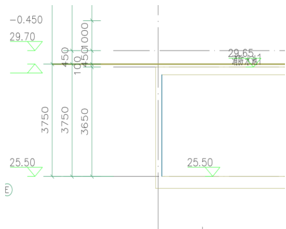
图 1.7 1#地下水池剖面图
