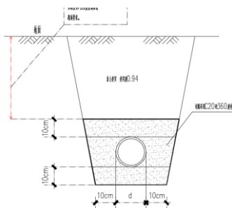
图 1.7 雨水管线大样图
