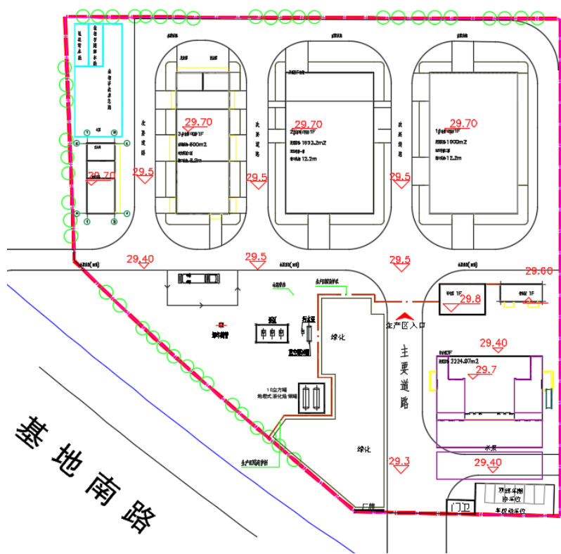
图 1.5 项目设计标高图
