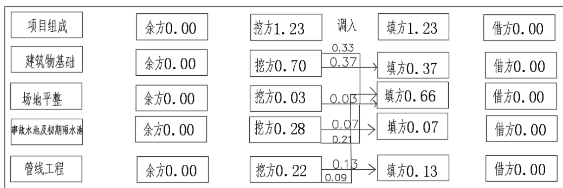
图 1.15 土石方平衡框图
