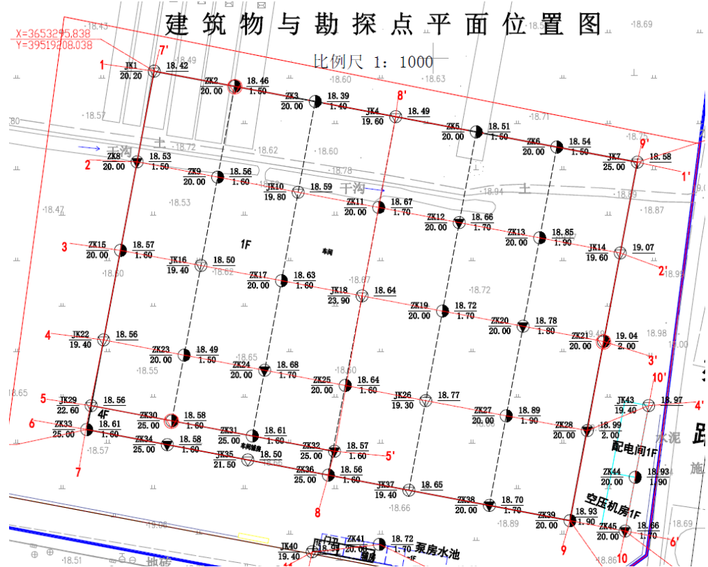
图 1.4 项目原始标高图
