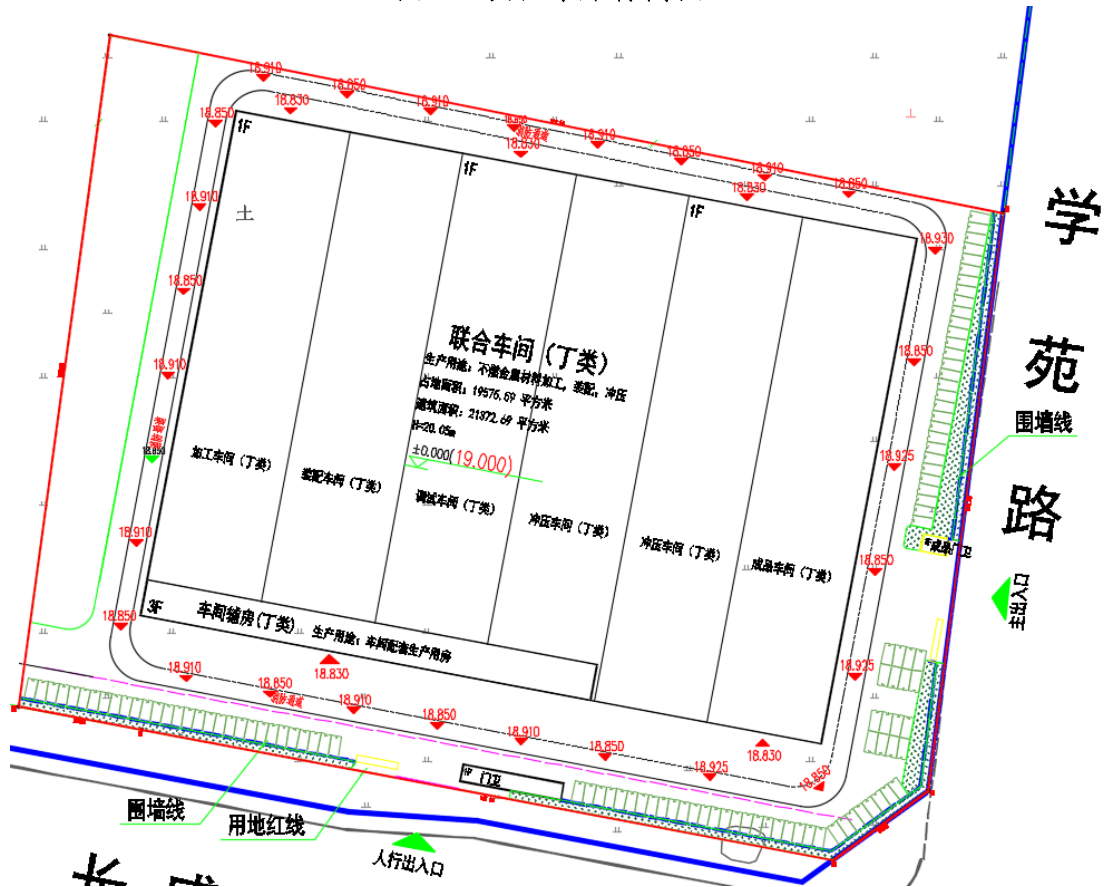
图 1.5 项目设计标高图
