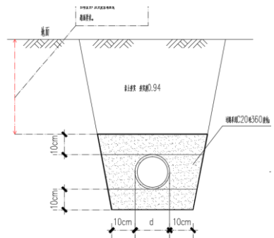
图 1.6 雨水管线大样图
