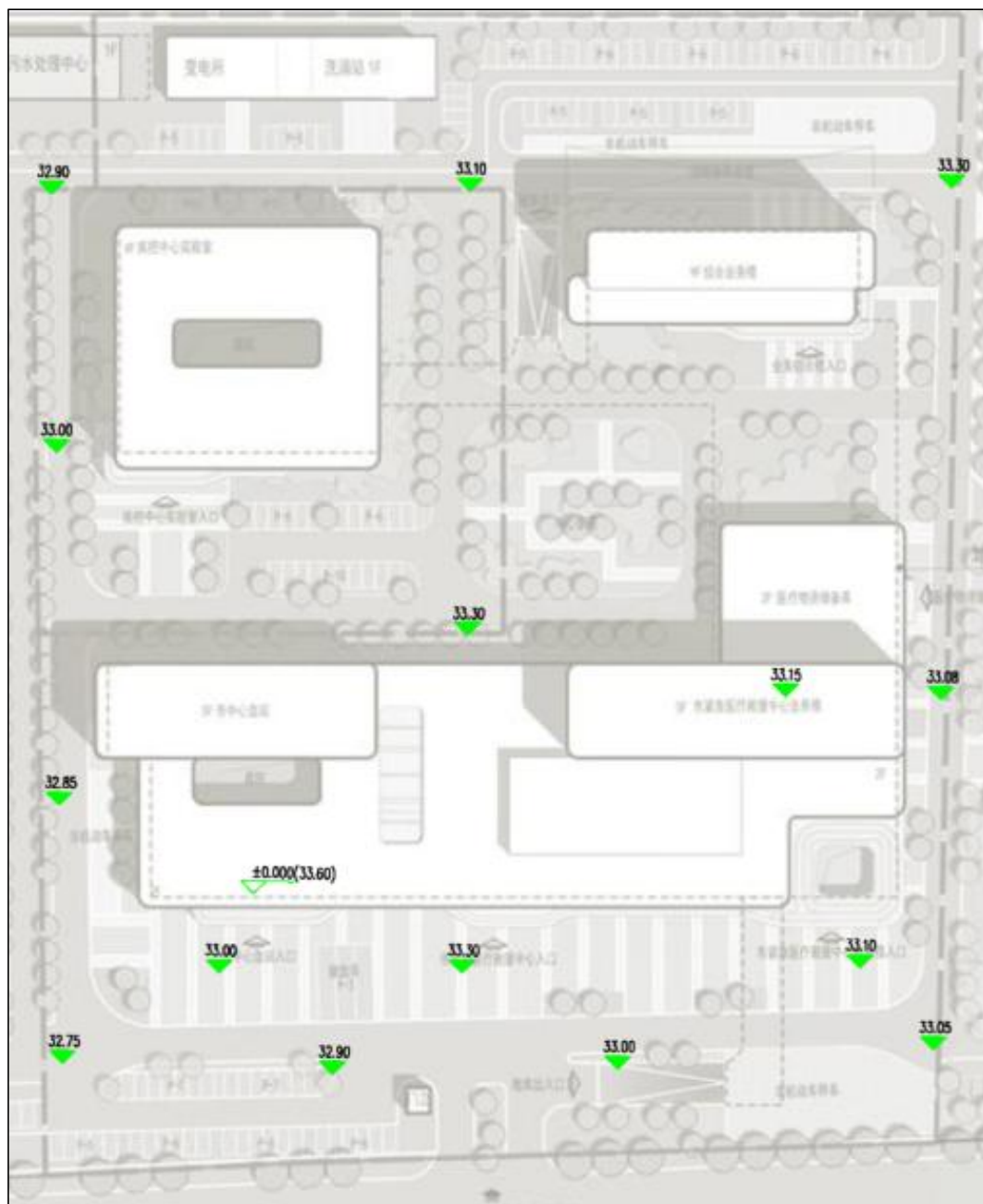
图 1.1-3 竖向标高
