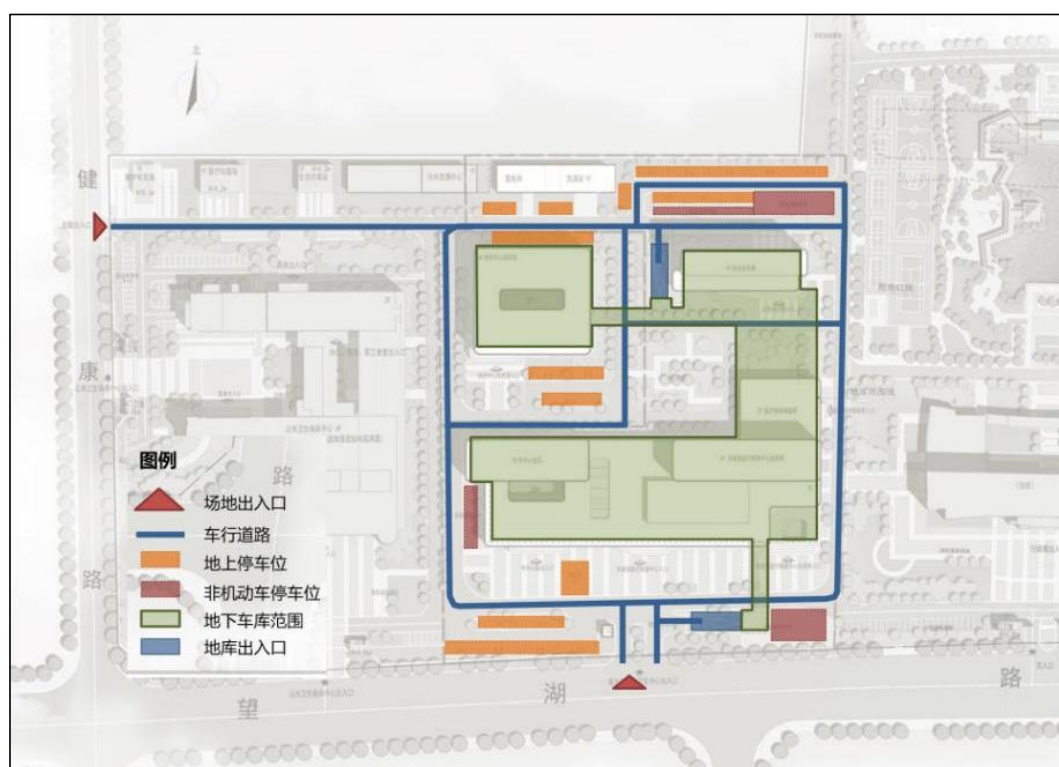
图 1.1-2 项目区道路、停车位、出入口布设图
