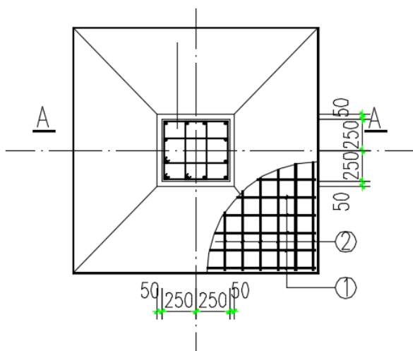
图 1.3 基准桩平面图
