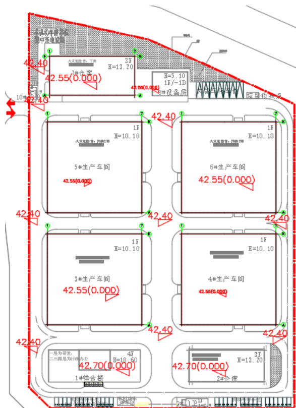
图 1.7 设计标高图
