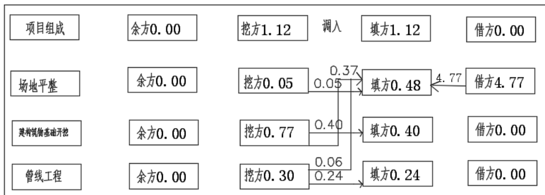
图 1.11 土石方平衡框图
