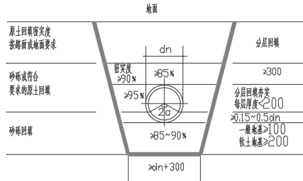
图 1.8 雨水管线大样图
