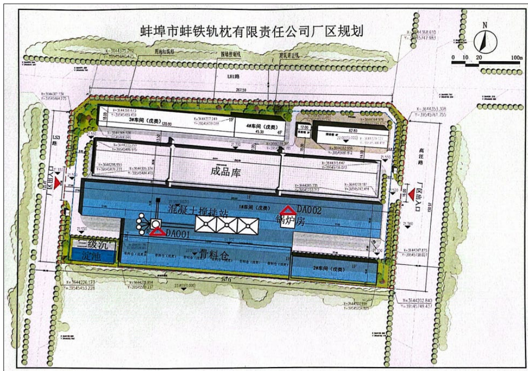
图 1.3-1 项目平面布置图
