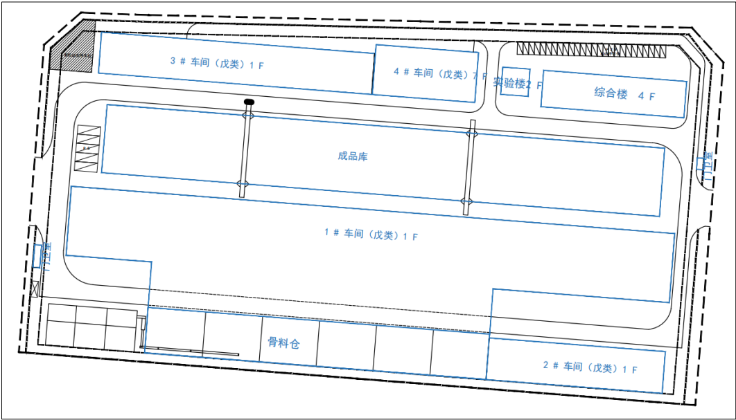
图 1.3-2 建构筑物布置图
