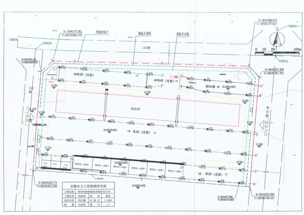
图 1.3-5 项目原地貌标高和设计标高对比图
