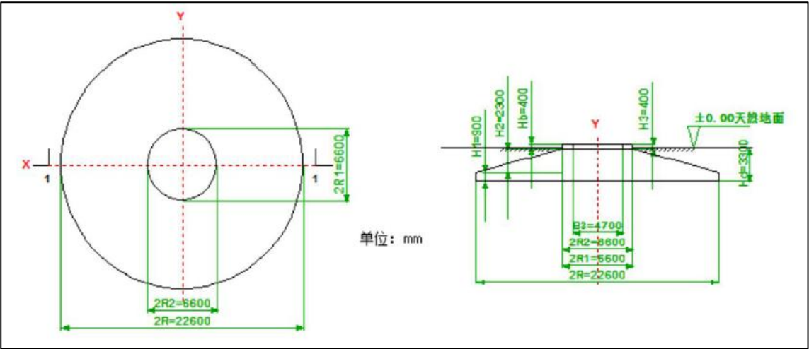
图 1.2 风电机组及箱变基础尺寸示意图
