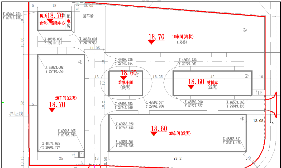
图 1.5 设计标高
