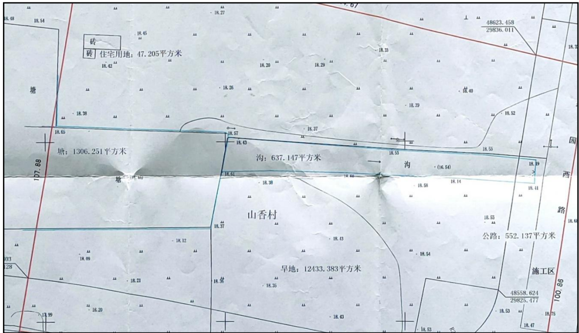
图 1.4 原始标高
