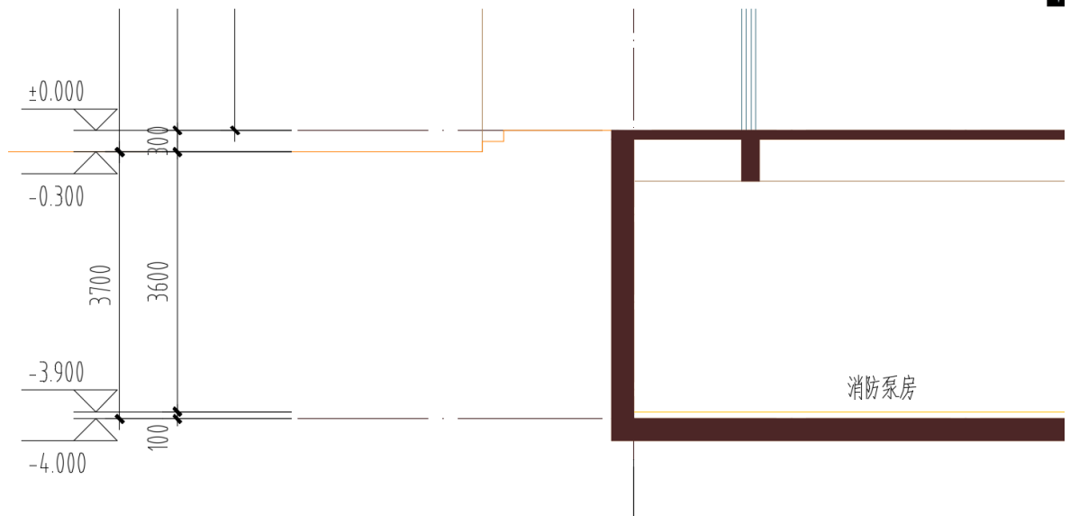
图 1.4 地库剖面图
