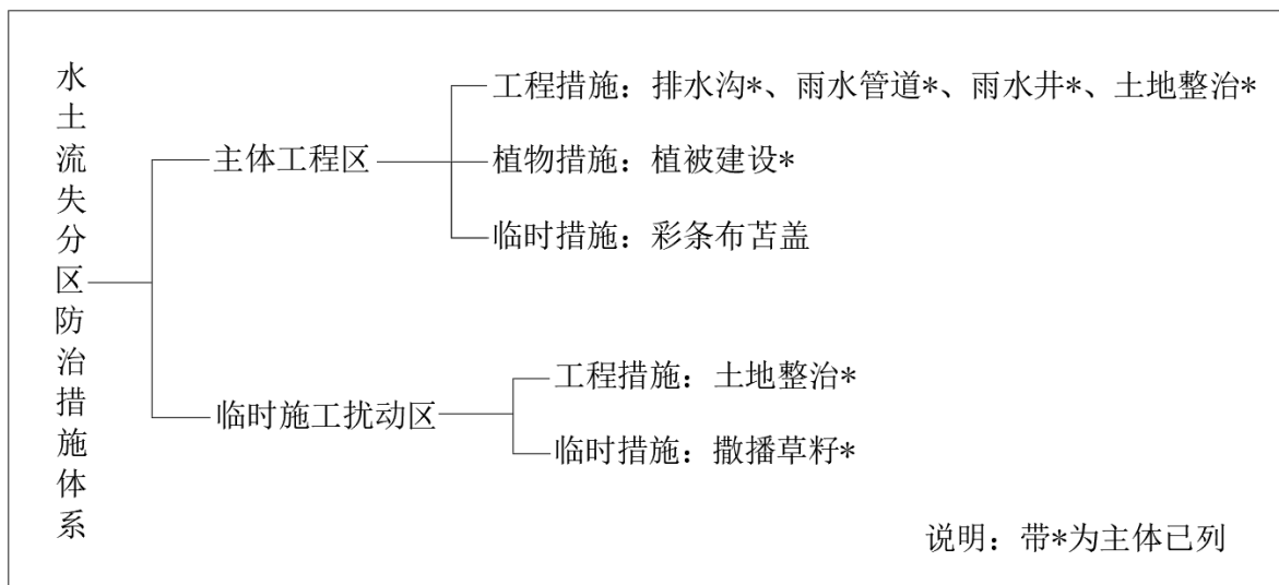
图 6.1 本工程水土流失防治体系框图
