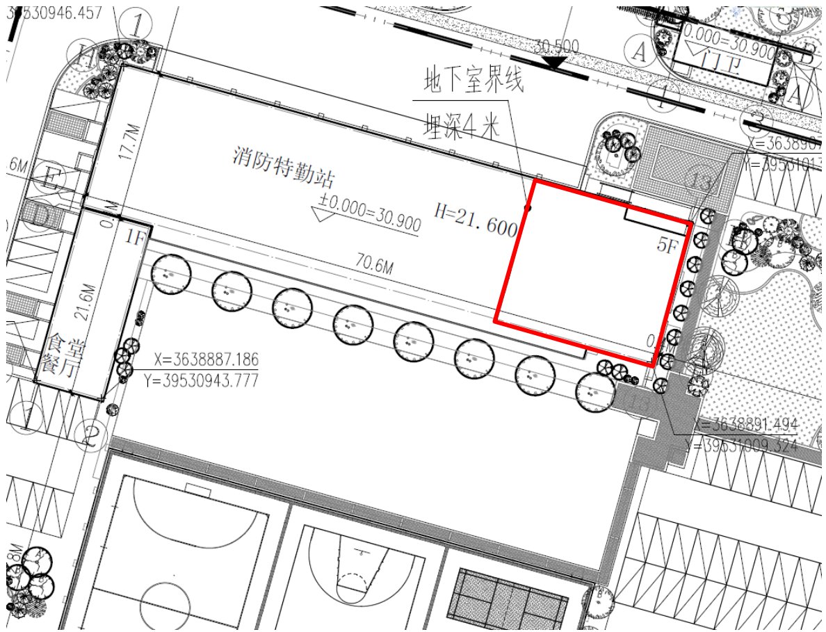
图 1.3 地下室范围分布图
